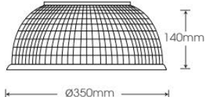
Chóa 90°
