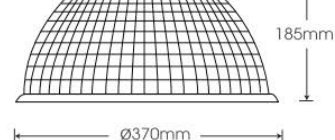
Chóa 45°
